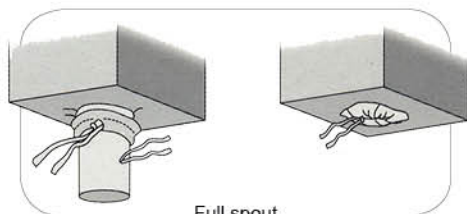
Full spout تخلیه با قیف حفاظت شده
