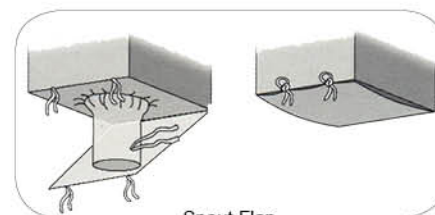
Spout Flap تخلیه با قیف و درپوش
